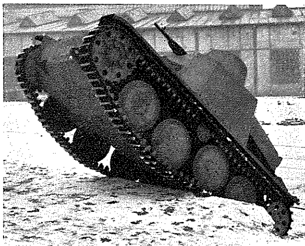
Let Kampvogn ved Overskridelse af 1 m lodret Mur lige før den »vipper ned«.
