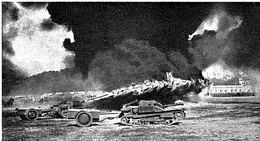
Italiensk Flammekaster-Kampvogn med tilkoblet Beholder, som medfører Brændstof. — Flammerne lader sig kaste over 30 m.
