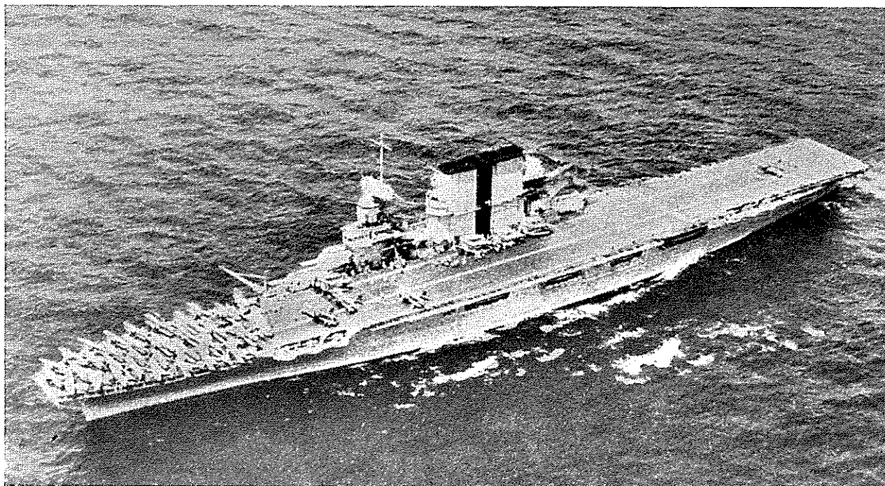
Amerikansk Aërodrømskib »Saratoga«. (Man bemærker Ø-Konstruktionen med 8 Stk. 20,3 cm Kanoner i 4 Dobbelttaarne).
