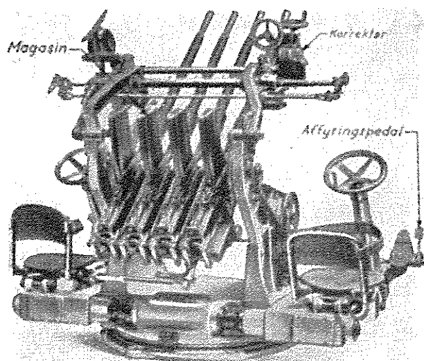
Fransk 13,2 mm Luftværnsmitrailleuse (Hotchkiss).
