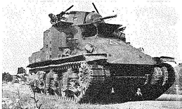
Middelsvær Kampvogn »General Grant«. Amerikansk Konstruktion.
