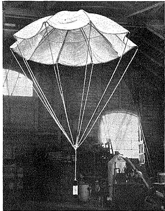
Lysbombe pr. Faldskærm. Bombebøssen er eksploderet og Lysbomben hænger i Skærmen.
