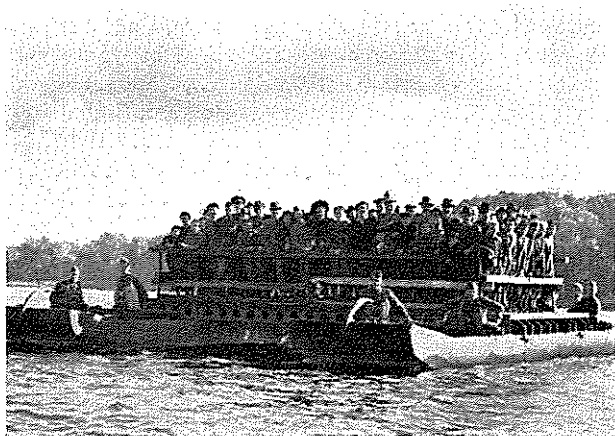
Nr. 7. Pontonfærge paa Djurgårdsbrunnsviken. (Fot. Pressens Bild)
