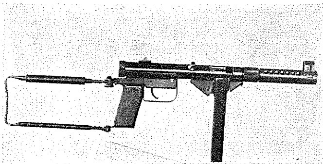
Fig. 3. 9 mm maskinpistol m/49.
