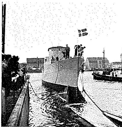
(8) Torpedobåd under afløbning. Den har netop forladt beddingen.
