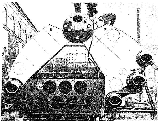
(9) Vandrørskedel til torpedobåd.
