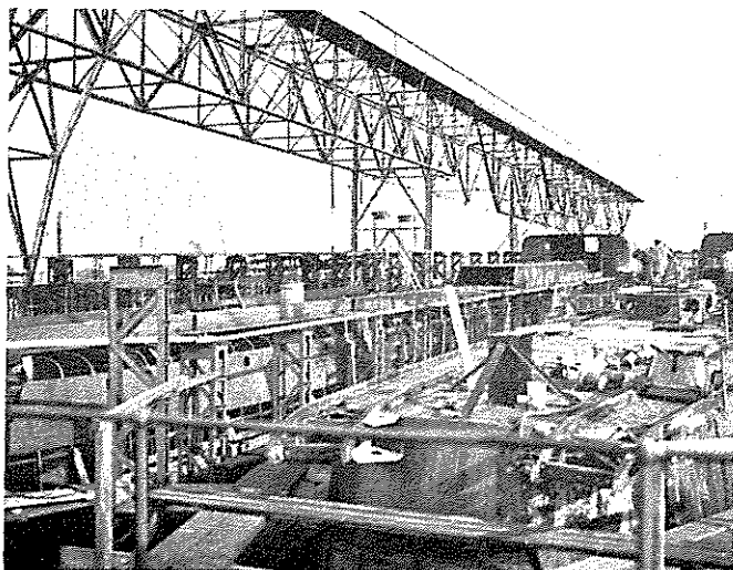
(6) To torpedobåde på huggebedding. Båden tilhøjre er snart klar til afløbning, medens båden tilvenstre er under opklædning.
