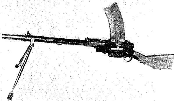
Fig. 4. 7.62 mm maskingevær m/48.
