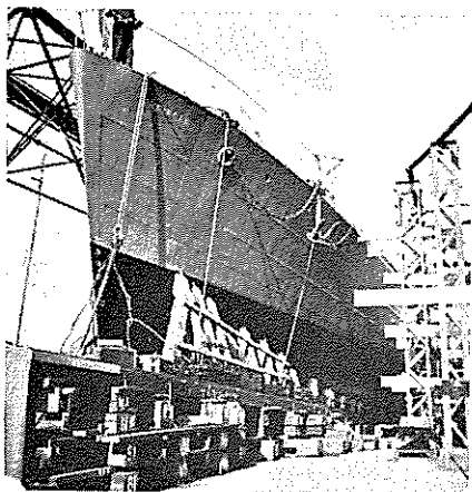
(7) Torpedobåd kort før afløbningen. Man ser afløbningsslæden og afløbningssbanen.
