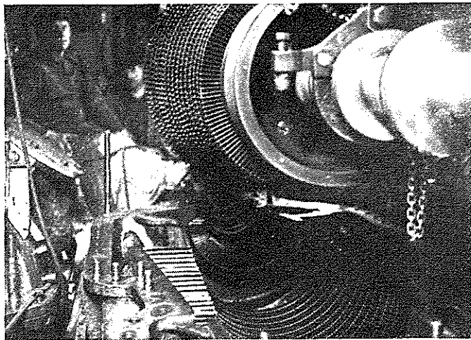
5 Damp turbine under montering. Rotoren med de mange turbine-skovle er ved at blive anbragt i turbinens underpart.
