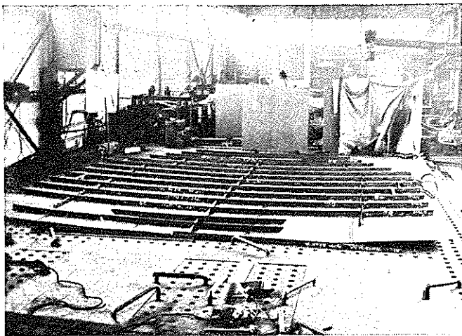
3 Færdigsvejst dæksparti med undersiden opad. Man ser svejtesømmene i pladerne og de påsvejste bjælker.
