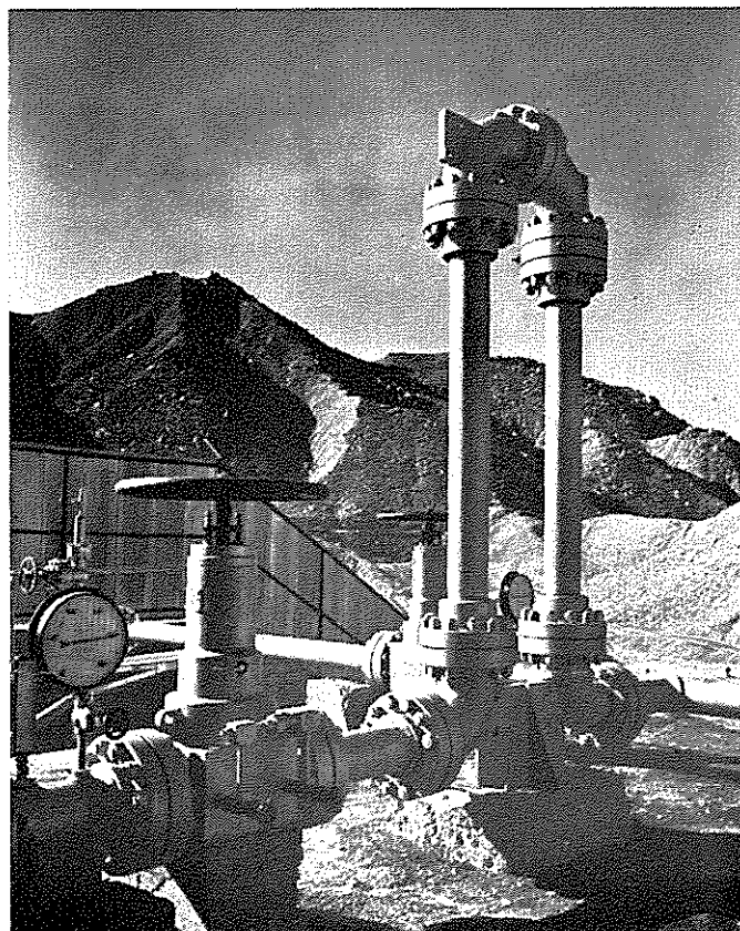
Oleströmmen fra de persiske kilder er altid blevet rationelt kontrolleret gennem det ventilsystem, som populært kaldes »juletræer«.
